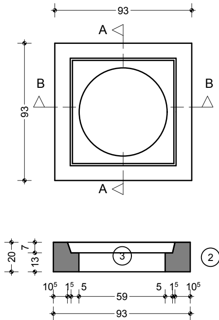
PIANTA COPERCHIO CARRABILE CON FORO DI ISPEZIONE CIRCOLARE
