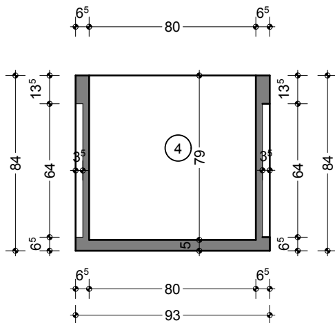
SEZIONE POZZETTO A-A SCALA 1:25
