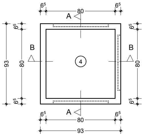
PIANTA POZZETTO SCALA 1:25
