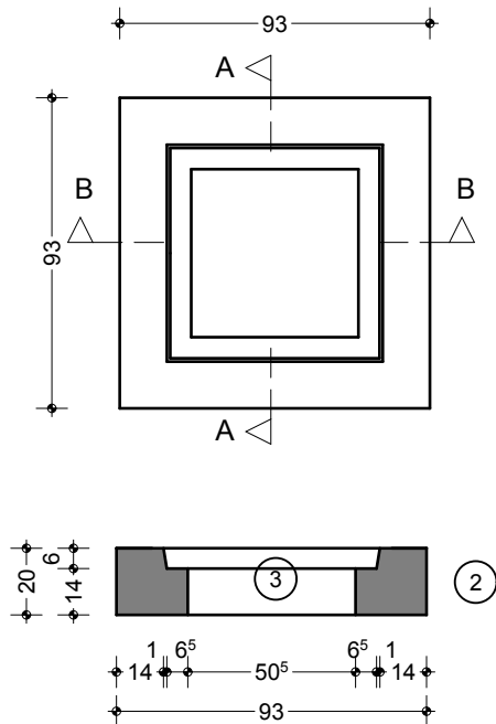
PIANTA COPERCHIO CARRABILE CON FORO DI ISPEZIONE QUADRATO
