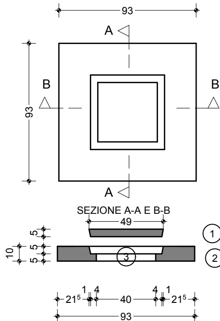
PIANTA COPERCHIO NON CARRABILE CON FORO DI ISPEZIONE QUADRATO
