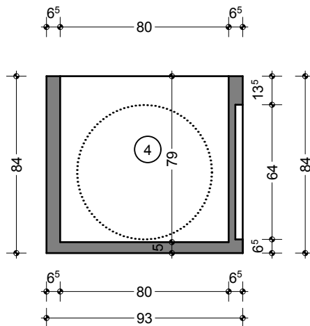
SEZIONE POZZETTO B-B SCALA 1:25
